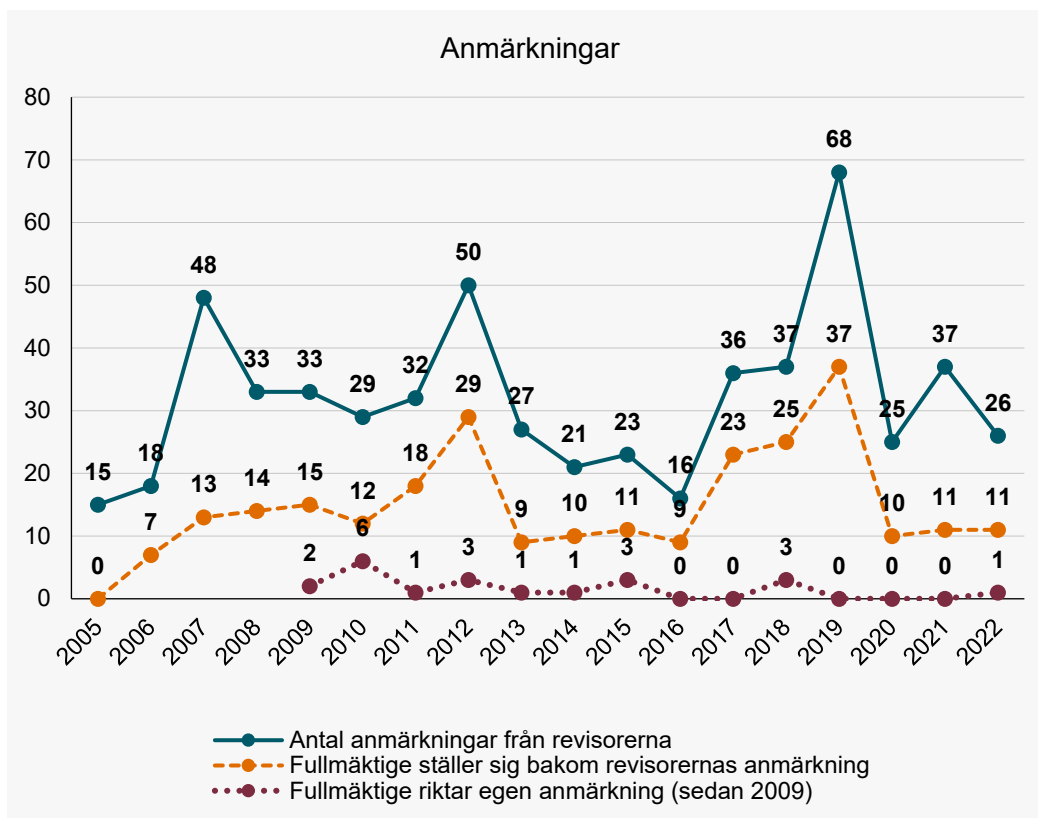
Diagram 1: Anmärkningar under 2005 - 2022
